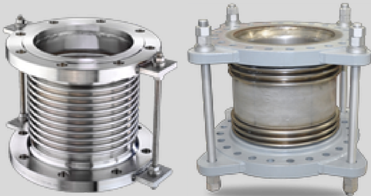
Metallic Rounded - TEJ, TMEJ & TUEJ,TUMEJ
